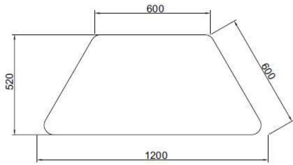
SEAT MODULE
