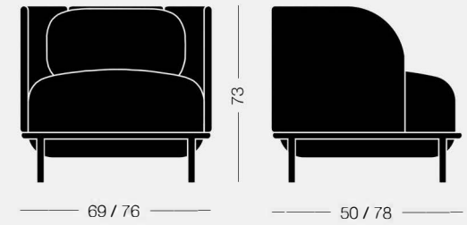
Bold 0C90 28,5 kg 0,50 m³ 1 pz Lounge chair, schienale basso Lounge chair, low backrest
